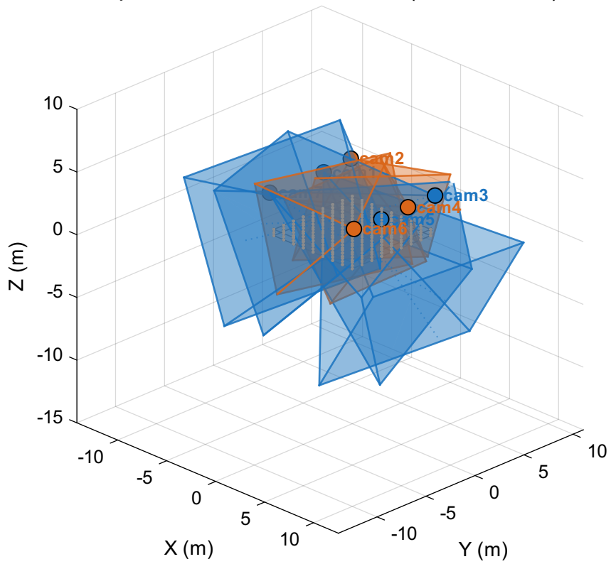
OptiTrack ad-hoc — 7 cams (Cost: 0.1449)
